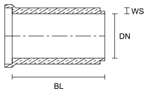
Version about mâle-femelle Ausführung mit Muffe und Spitzende uniquement en type lourd
