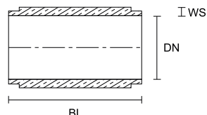
Version about mâle-mâle Ausführung Spitz-Spitz ausschliesslich in Typ lourd erhältlich
