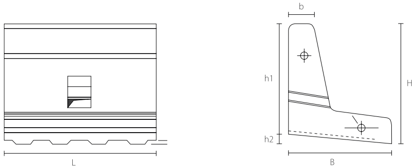
Bouteroue avec ou sans trou de drainage / Prellstein mit oder ohne Entwässerungsloch
