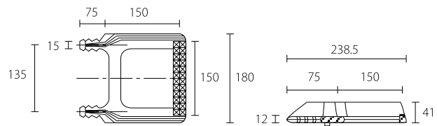
Etriers DIN 1212 E à enfoncer Steigeisen DIN1212 E einschlagbar
