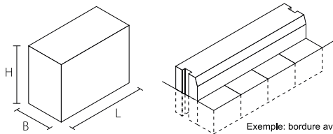
Exemple: bordure avec pavés pour fil Beispiel: Bordstein mit Rinnenpflastersteinen
