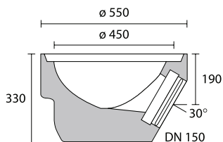
Base DN 150 / Boden DN 150 DIN 4052-1a
